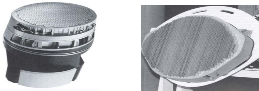
Рисунок 1. – АФАР AMSAR и AN/APG-77 бортовых РЛС тактической авиации
