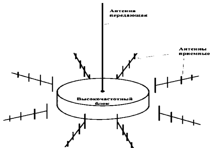
Рисунок 1. - Высокочастотный блок моноимпульсной РЛС
