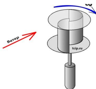
Рисунок 3. – Ротор Савониуса
