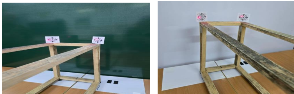
Рисунок 3. – А, В - Демонстрация точности фиксации угловых изменений положения конструкции
