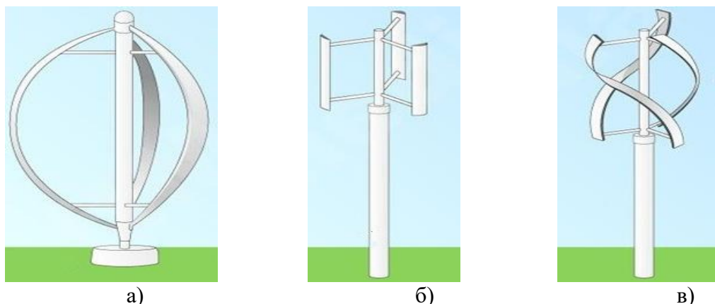
Рисунок 2. – а) Ротор Дарье, б) Ротор Дарье типа Н, в) винтообразный ротор Дарье
