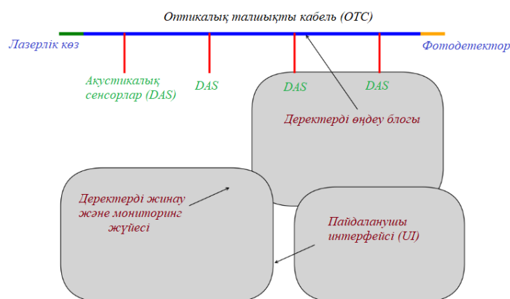
3-сурет. – Оптикалық талшықты технологиялар негізінде таралған акустикалық сенсорларды қолдану құрылымдық сұлбасы
