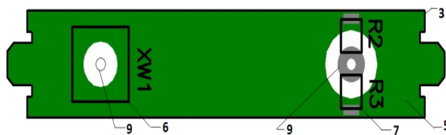
Рисунок 4 а. – Вид внешней стороны одного из отрезков двустороннего ламината с подключением нагрузочного резистора
