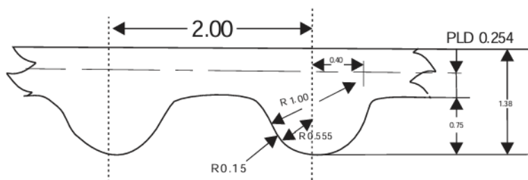
Рисунок 1. – Проектирование узлов осей 3-D принтера
