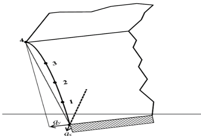
Рисунок 2. – Крен ребра здания
