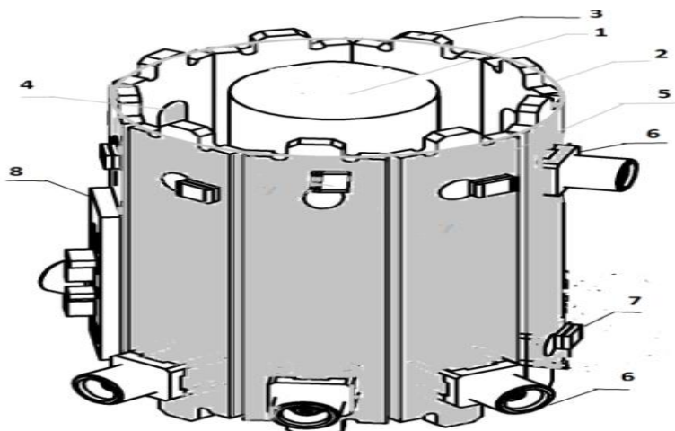
Рисунок 3. – Внешний вид коаксиального направленного ответвителя
